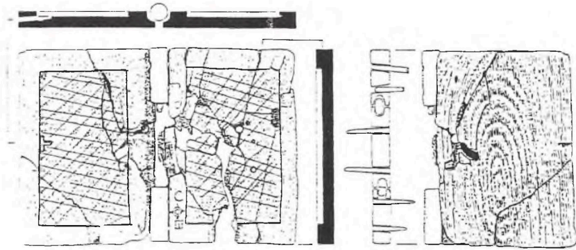
Şekil 2. Uluburun Balmumu Yazı Takımı. Menteşe düzeni, eksik olan menteşe ve ağaç çivileri ile birlikte. (Çizim: Neita Piercy). (Payton, 86, 1991).
